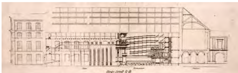
Abb. 9: Das kurfürstliche Opernhaus im Mannheimer Schloss, Längsschnitt, o. J.
