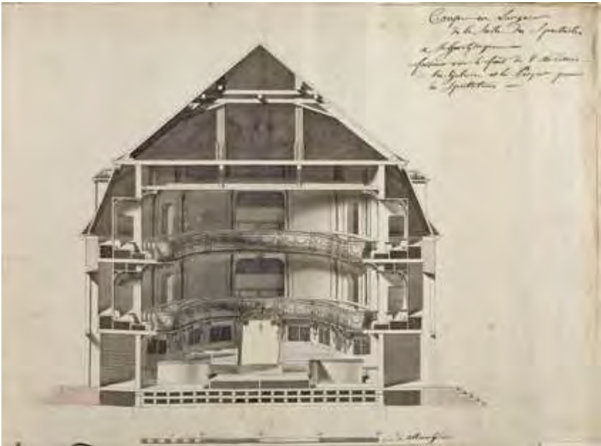
Abb. 14: Nicolas de Pigage: Schwetzingen, Theater, Querschnitt durch den Zuschauer- raum, um 1755.
