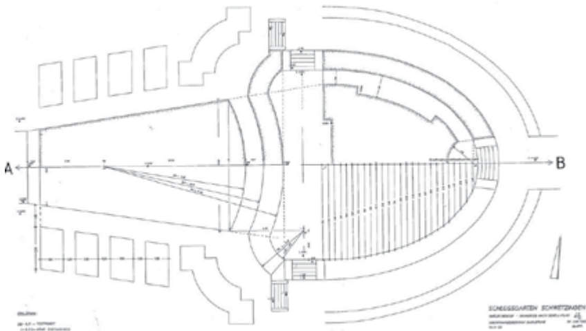
Abb. 68: Hubert Wolfgang Wertz: Grundriss des Naturtheaters nach dem Plan von Nicolas de Pigage, 1783, und Grabungsfunden, Massstab 1:50.
