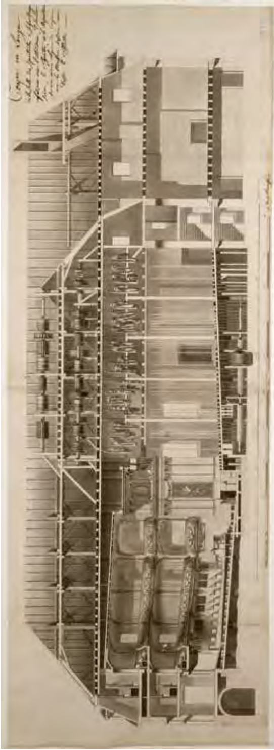
Abb. 13: Nicolas de Pigage: Schwetzingen, Theater, Längsschnitt, um 1755.
